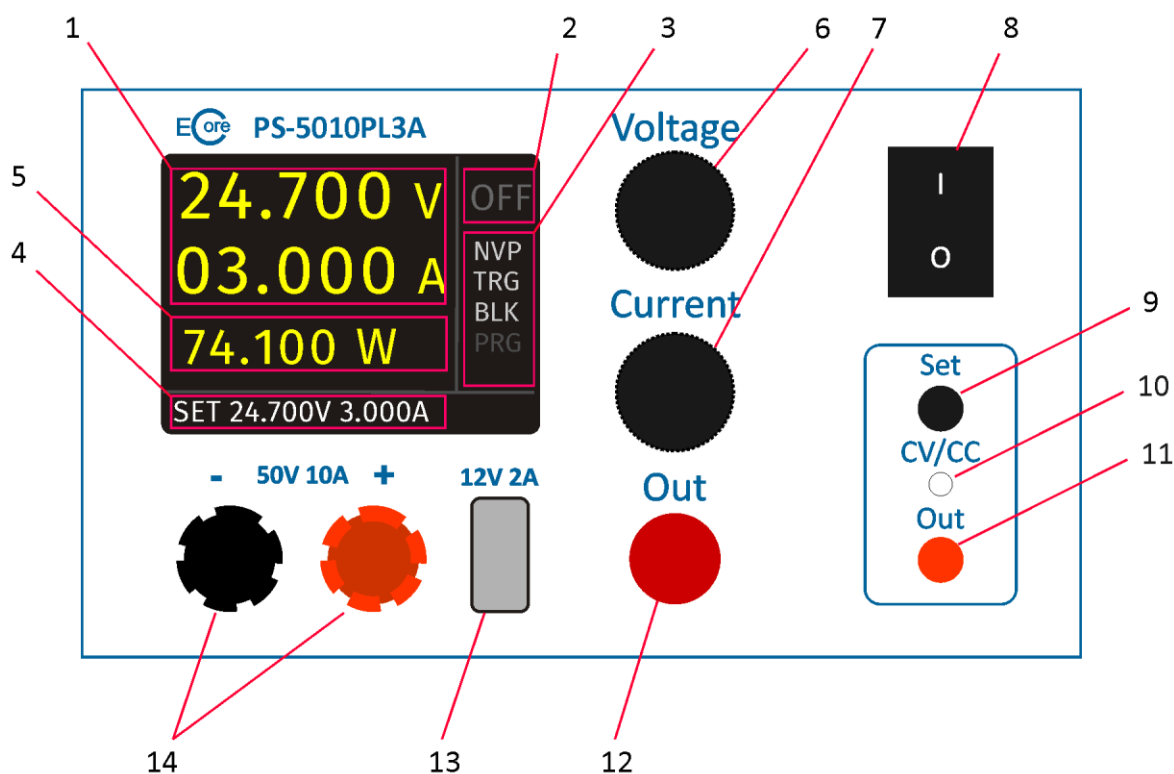
Рисунок 1 – внешний вид лицевой панели
