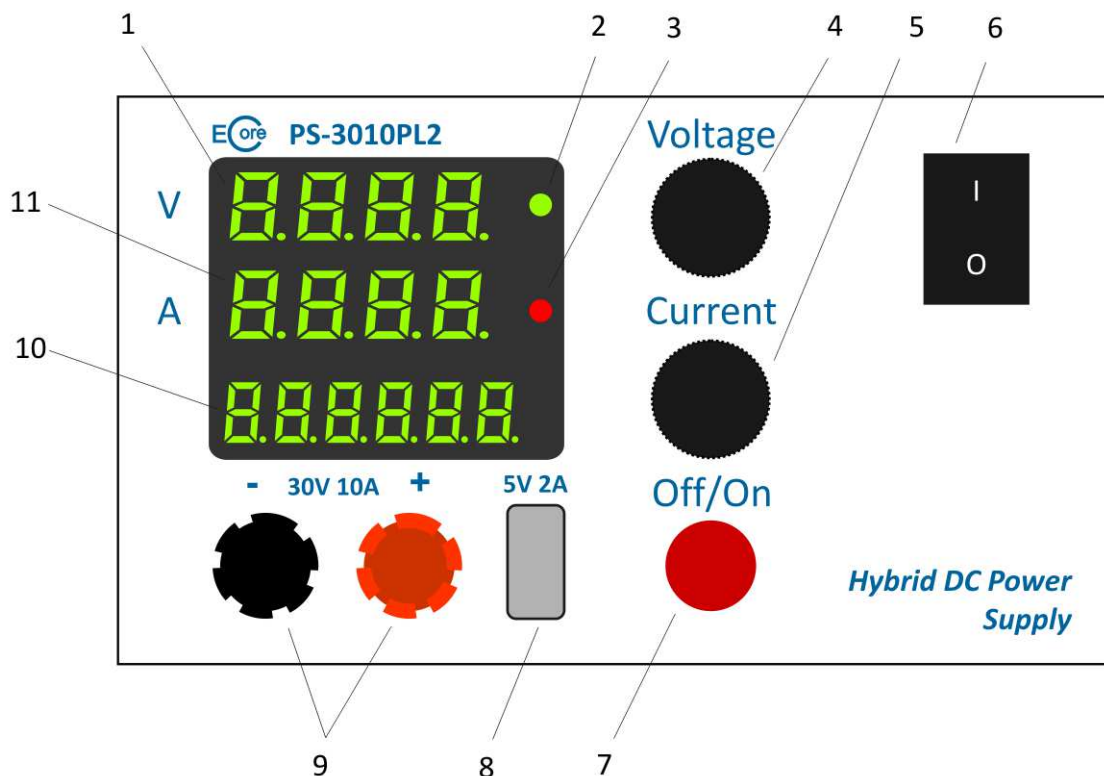
Рисунок 1 – внешний вид лицевой панели
