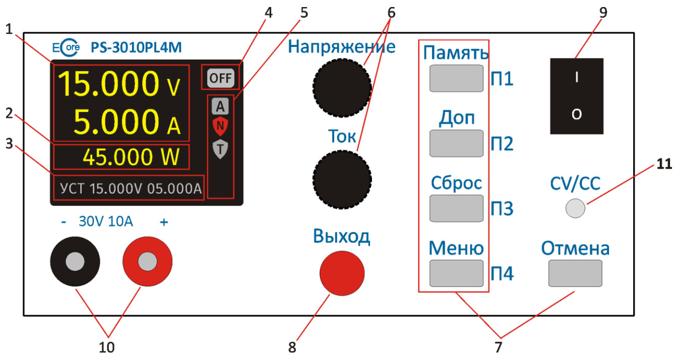
Рисунок 1 – внешний вид лицевой панели
